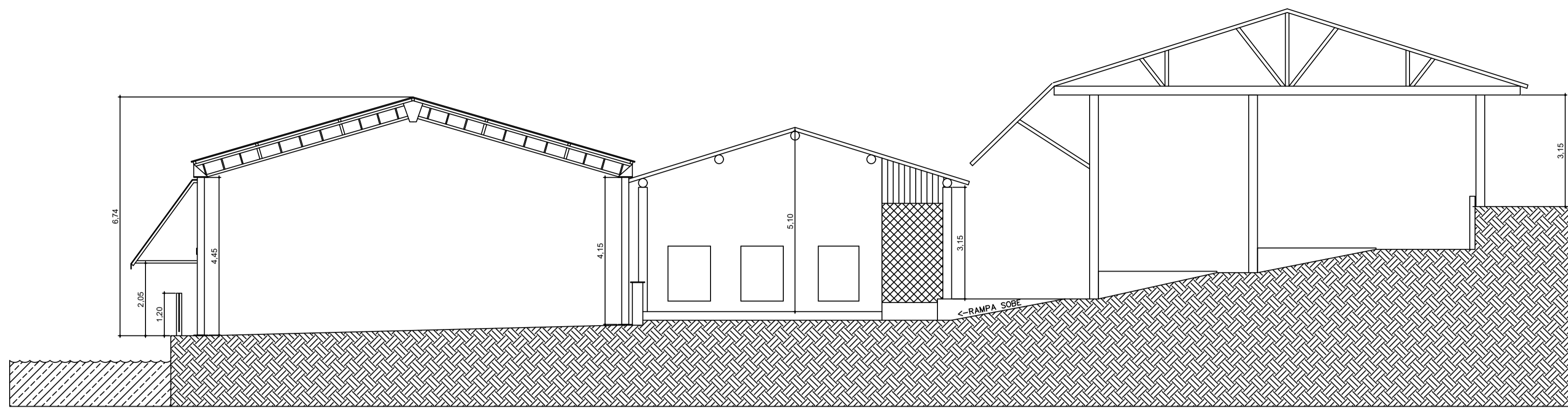
CASA DO LAGO - CORTE AA Esc.: 1:100
